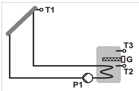
Schemat 2 - ładowanie zasobnika z kolektora słonecznego i dogrzewanie zasobnika grzałką.
