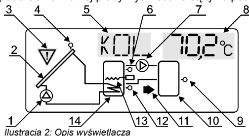
Ilustracja 2: Opis wyświetlacza
