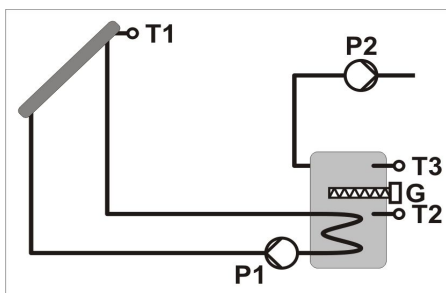
Schemat 3 - ładowanie zasobnika z kolektora słonecznego i zrzut nadmiaru ciepła.
