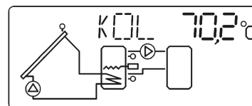
Ilustracja 5: Schemat wyświetlany przez regulator przy pracy ze schematem 4.
