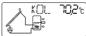
Ilustracja 4: Schemat wyświetlany przez regulator przy pracy ze schematem 3.
