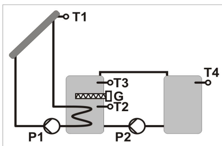
Schemat 4 - ładowanie zasobnika z kolektora słonecznego i przepompowywanie ciepła do drugiego zbiornika (na zasadzie różnicy temperatur).
