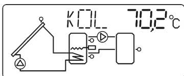
Ilustracja 6: Schemat wyświetlany przez regulator przy pracy ze schematem 5.
